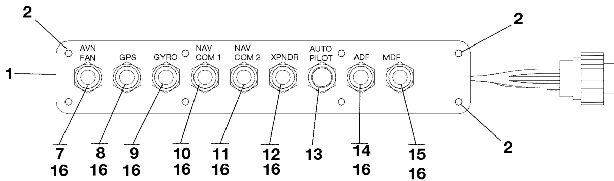
VIEW A-A
