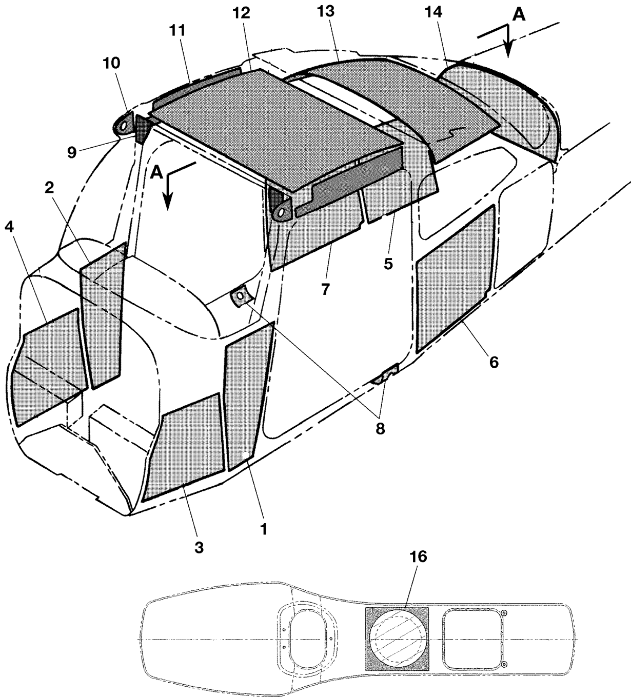
VIEW A-A
