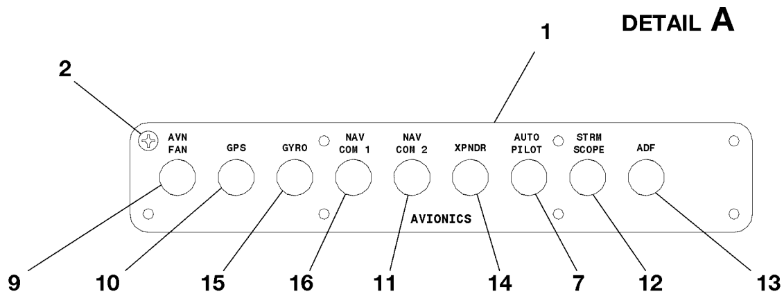
VIEW A-A
