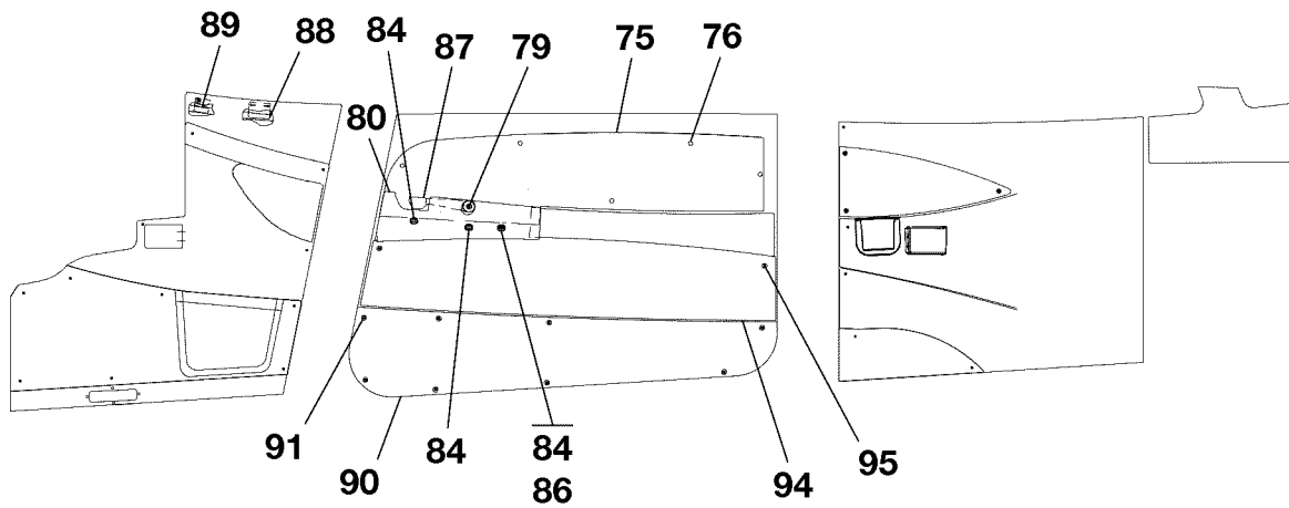
VIEW A-A
