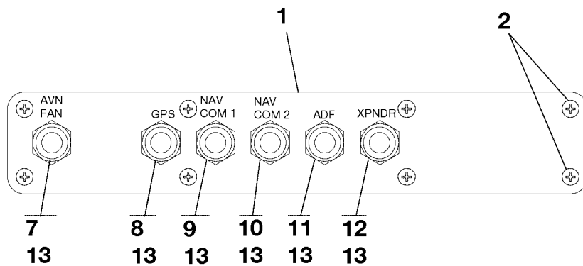
VIEW A-A
