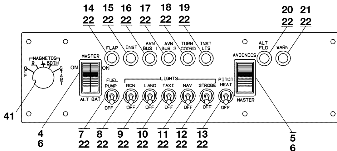
VIEW A-A
