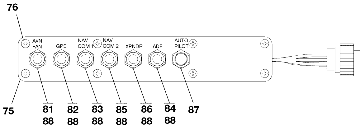
VIEW A-A
